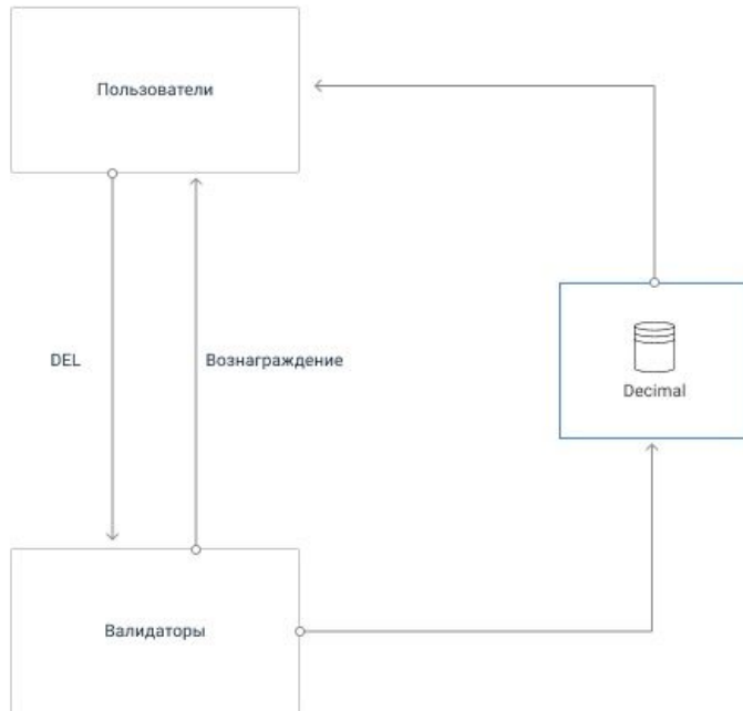
Рис. 5 - делегирование.
